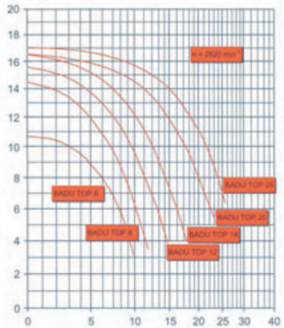
Q (m 3 /h) - Badu Top S
