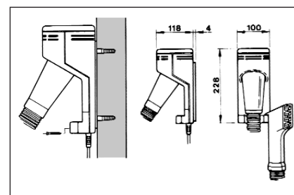
Mise en marche et arrêt automatique par simple décrochage de la buse
