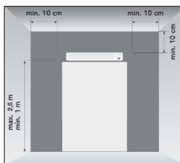
Hauteur installation
