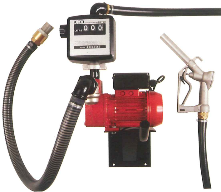
Référence JEV1033 en monophasé avec compteur Référence JEV1133 en triphasé avec compteur
