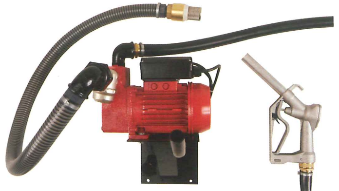
Référence JEV10EQ en monophasé sans compteur Référence JEV11EQ en triphasé sans compteur
